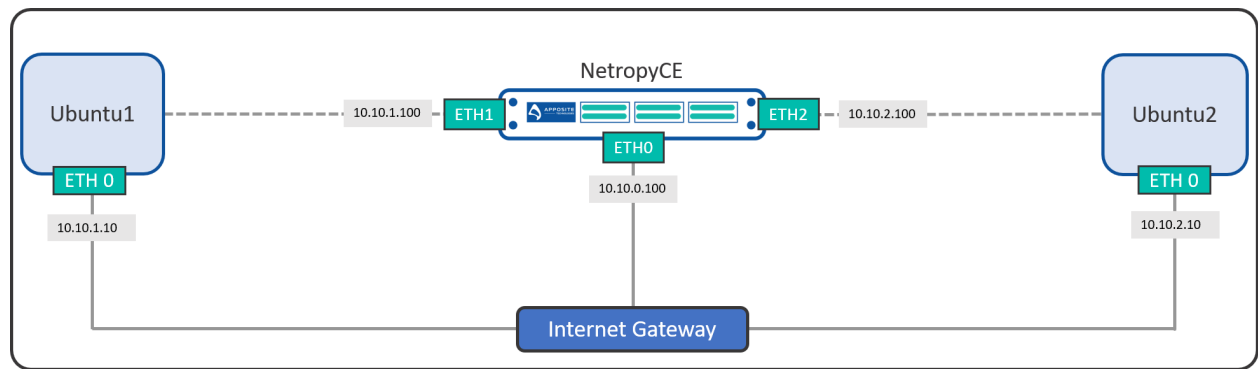
AWS VPC 10.10.0.0/16
