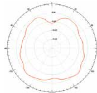
0° E-Plane
