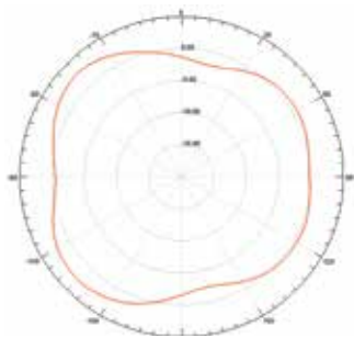
45° H-Plane
